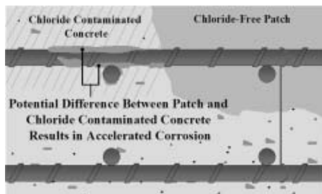
Fig. 1—“Ring-anode” corrosion.
